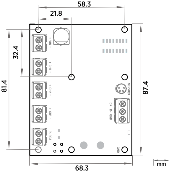
Figura 18 Dimensões da placa de componente do HMM170
