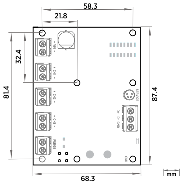
図 22 HMM170 回路基板寸法
