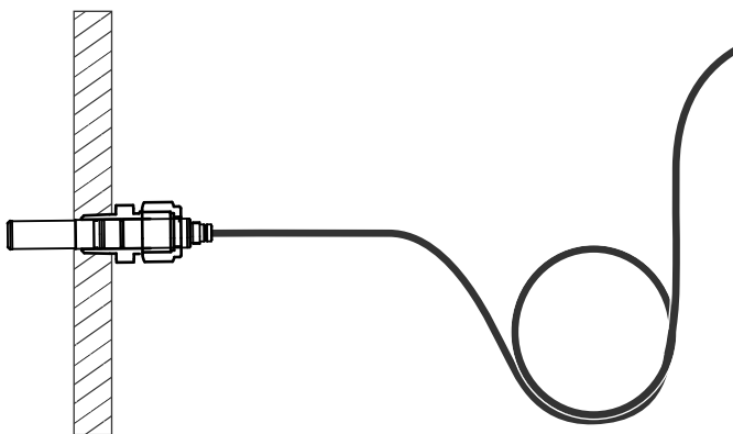
Figura 16 Instalación de la sonda HMM170 en una pared
