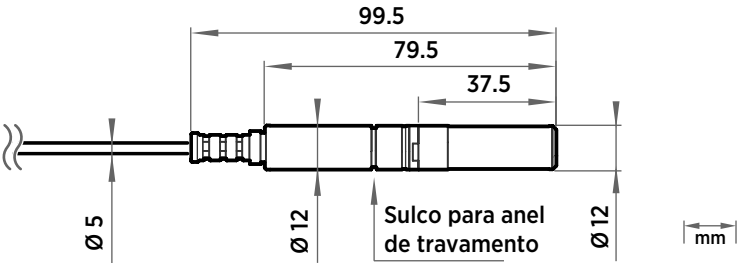
Figura 17 Dimensões da cabeça da sonda HMM170
