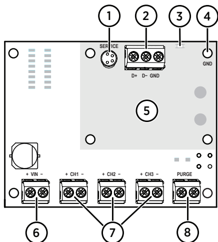
图 27 HMM170 电路板
