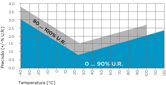
Precisão da medição de umidade da HMP9 como uma função da temperatura
