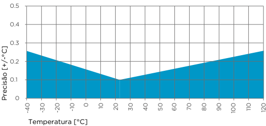
Precisão da medição de temperatura da HMP9 em todo o alcance
