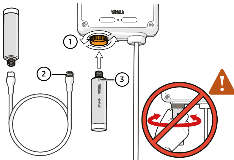
図 19 プローブとケーブルのIndigo200への取り付け
