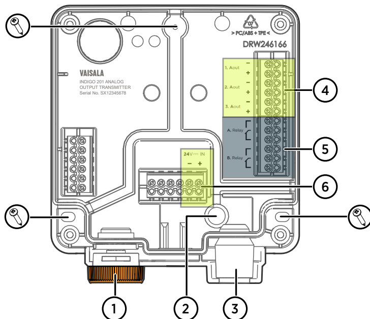
图 24 Indigo 201 数据处理单元基座主部件和安装螺钉位置
