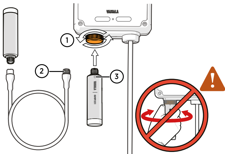
图 26 将探头和电缆连接到 Indigo200
