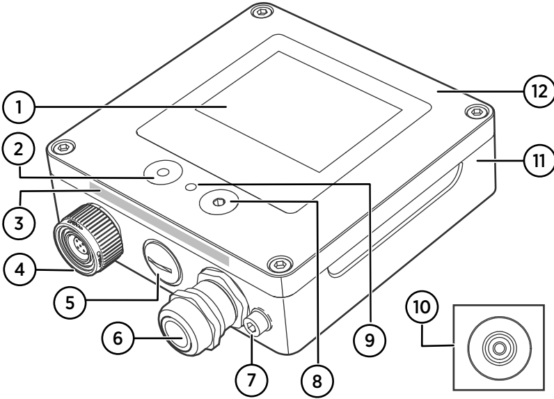
图 62 Indigo300 数据处理单元部件
