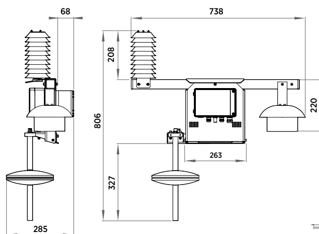
Dimensões do Indigo500MIK com kit de montagem na parede
